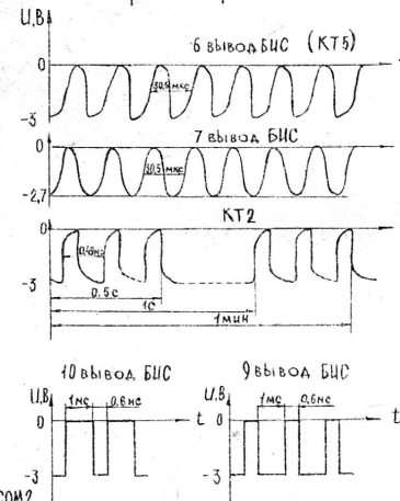
Эпюры напряжений
